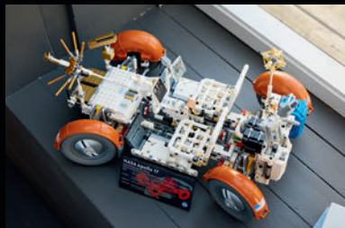
42182 NASA Apollo Lunar Roving Vehicle - LRV Le véhicule d'exploration lunaire NASA Apollo - LRV 18+ years / ans
